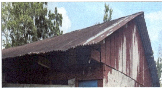
Fotografía 5: Vista de la estructura de techo y cubierta de lámina, se instalará estructura de metal galvanizada y cubierta de lámina troquelada Cal 26.
